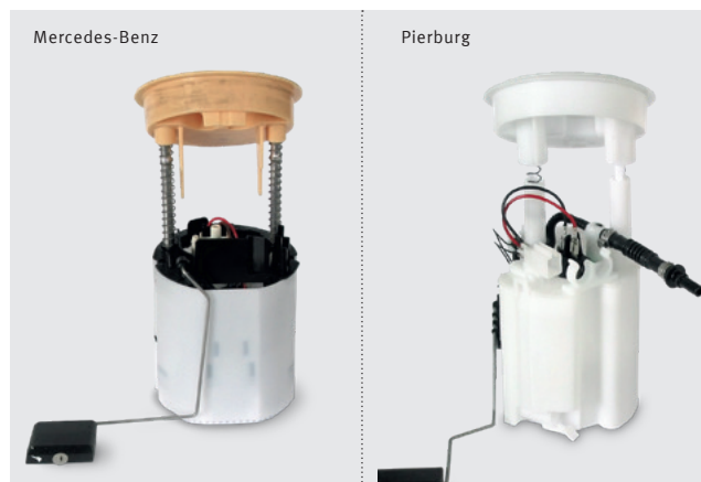
Fig. 1: Moduli alimentazione carburante a confronto
