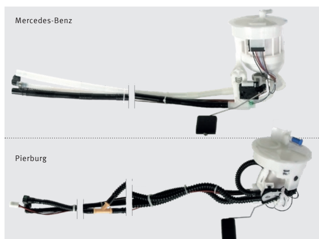
Fig. 2: Trasduttori di livello carburante a confronto
